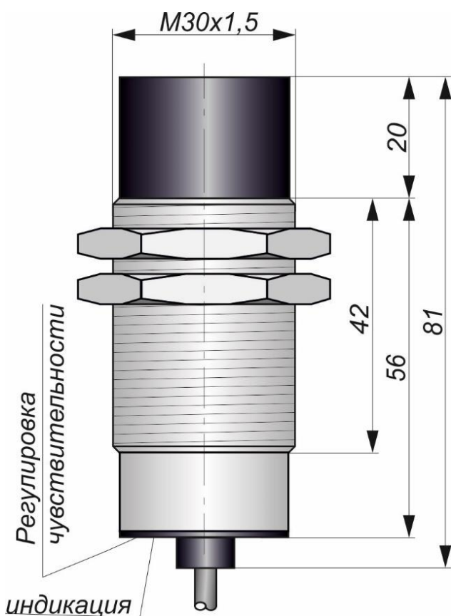
Габаритный чертеж
