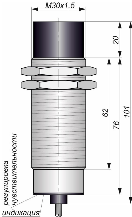
Габаритный чертеж
