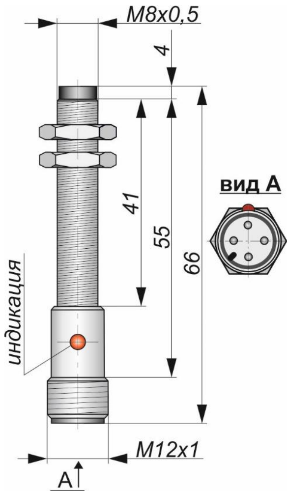
Габаритный чертеж
