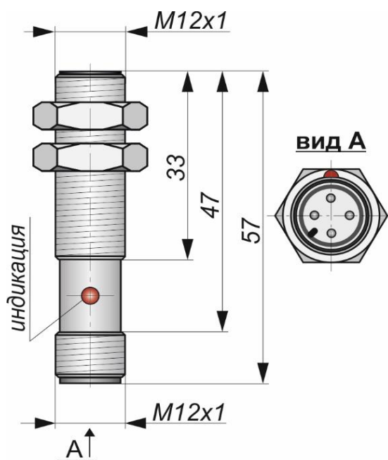
Габаритный чертеж
