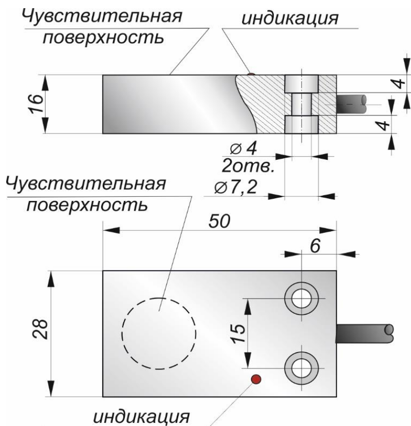
Габаритный чертеж
