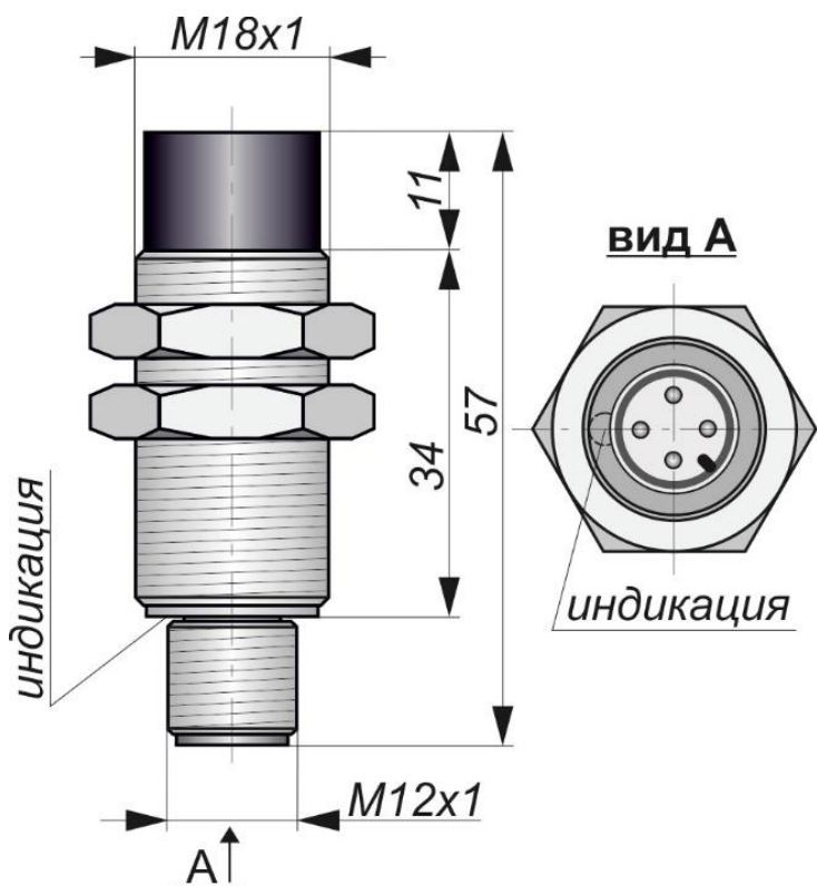
Габаритный чертеж
