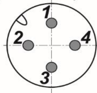
Цоколевка разъема
