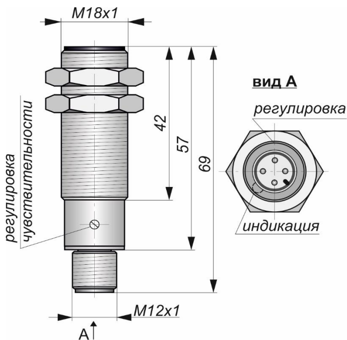
Габаритный чертеж
